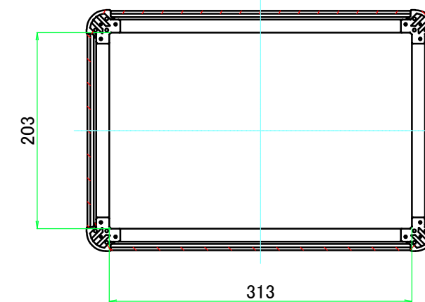
C-C ( 1 : 5.5 )
