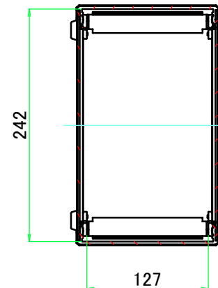
A-A ( 1 : 5.5 )
